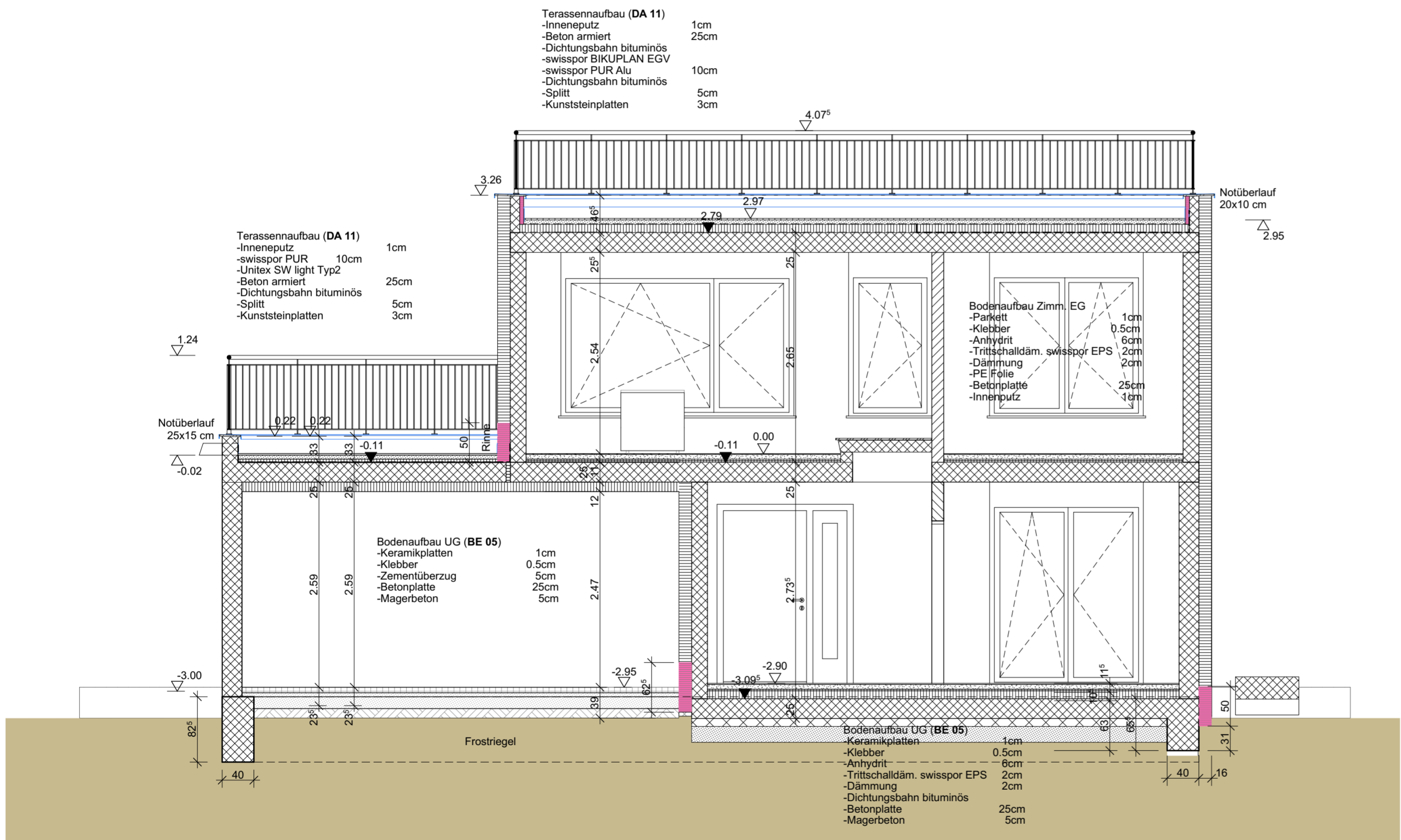
SCHNITT D_D
